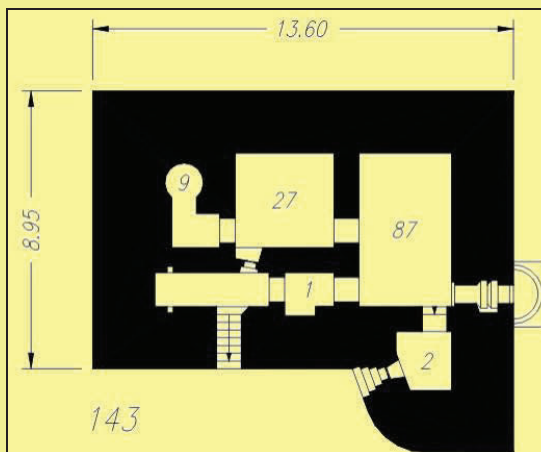
1: gasluuis; 2: nabijverdediging; 87: ruimte voor 6 manschappen; 27: rekenkamer; 9: observatiekoepel.
