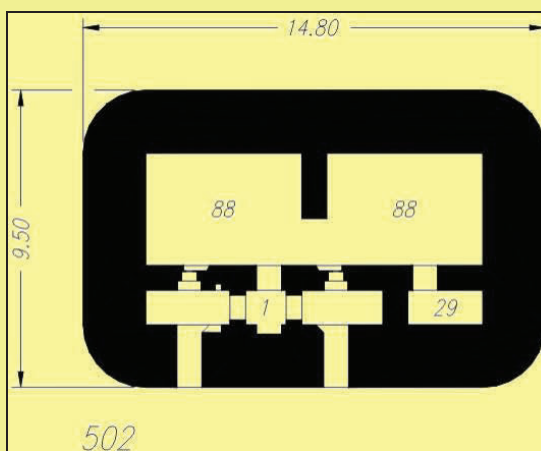
1: gasluuis; 88: ruimte voor 10 manschappen; 29: voorraadruimte.
